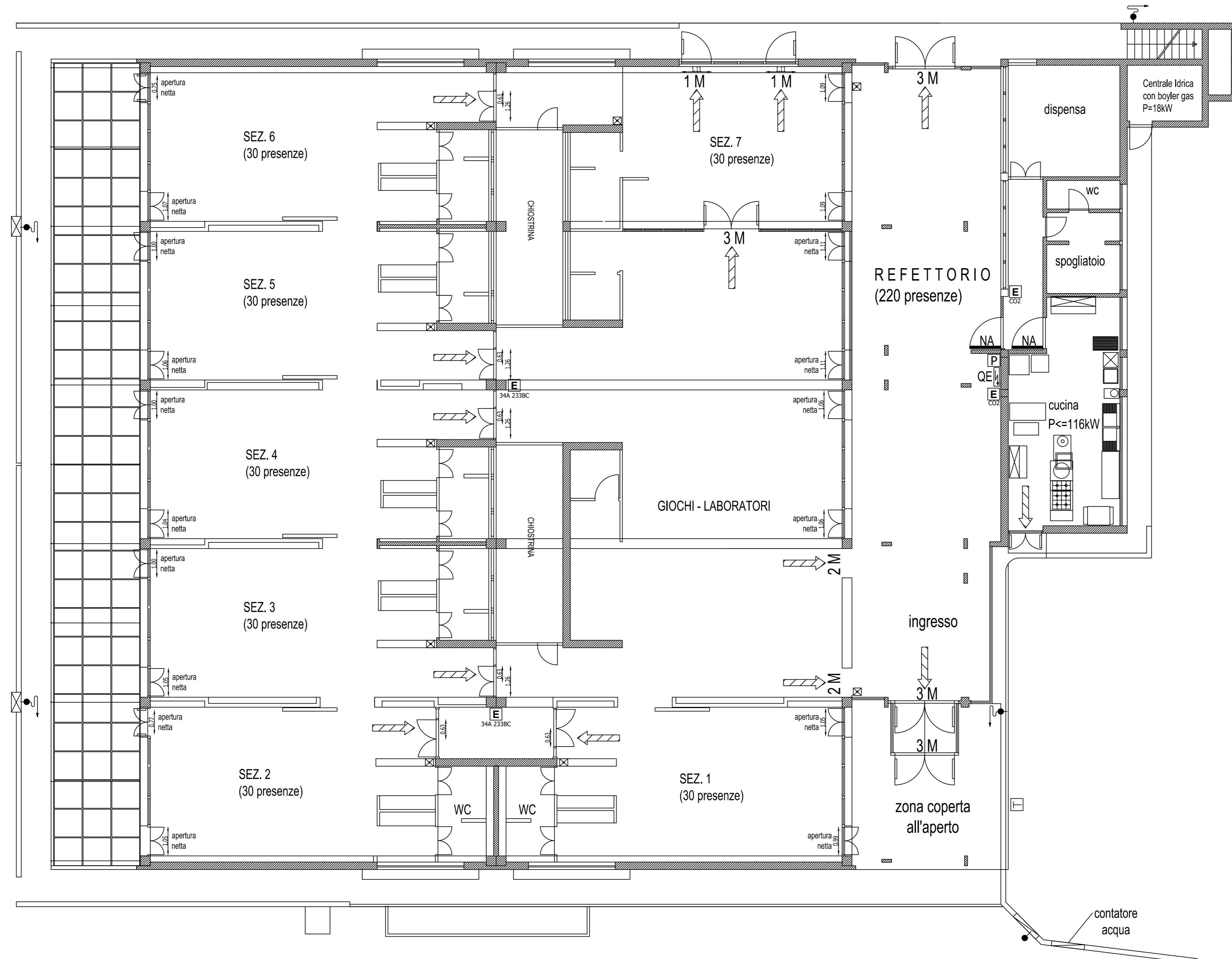
PIANTA PIANO TERRENO - STATO ATTUALE
